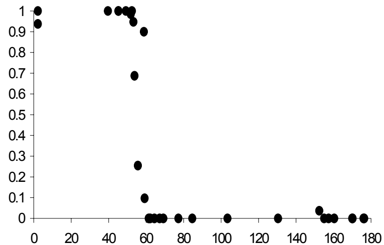
Emd
