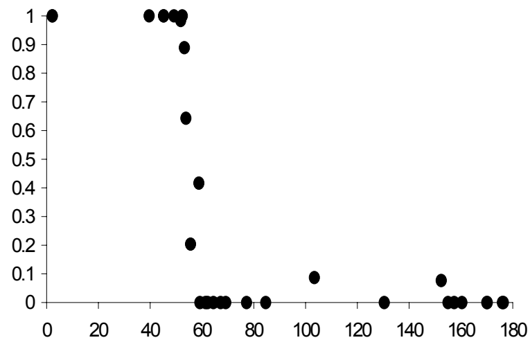
DXMit18.2
