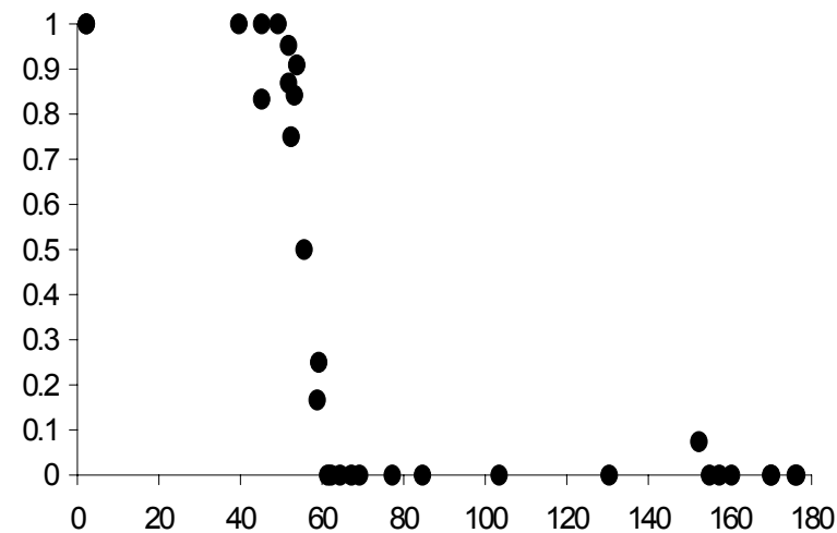
Sep6b
