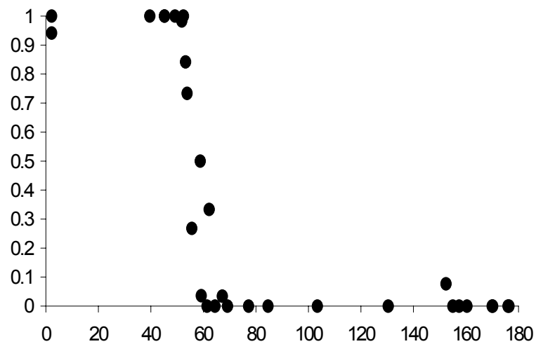
Trpp5
