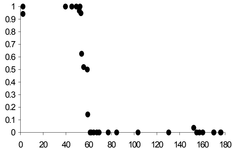
Pou3f4
