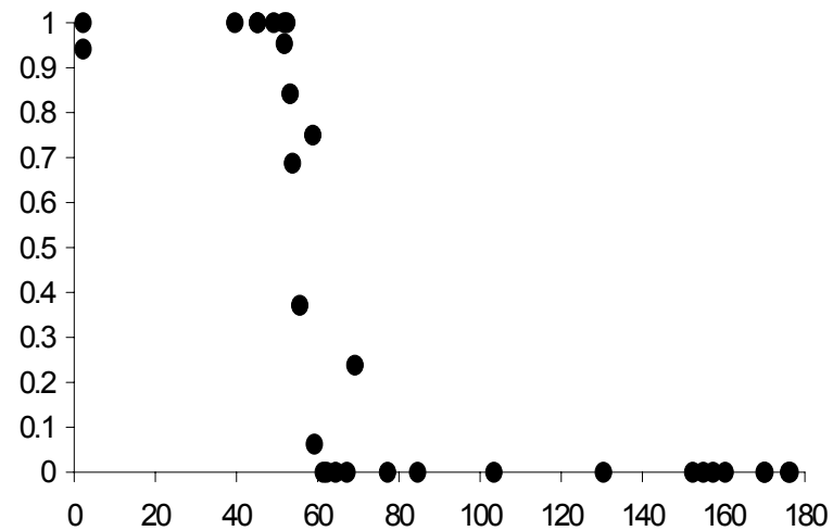
Nt
