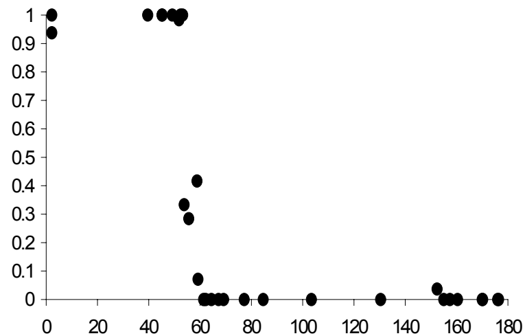
Pola1
