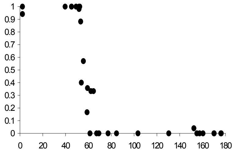
Btk2
