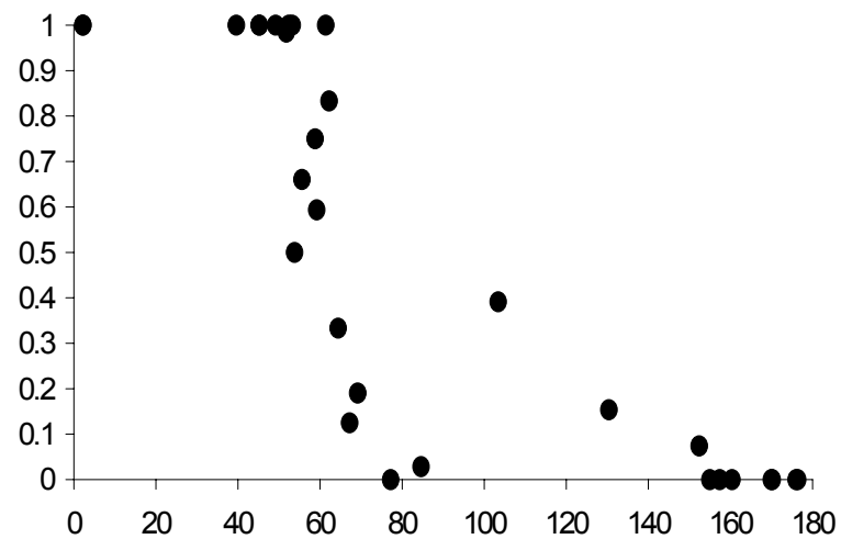
Plp
